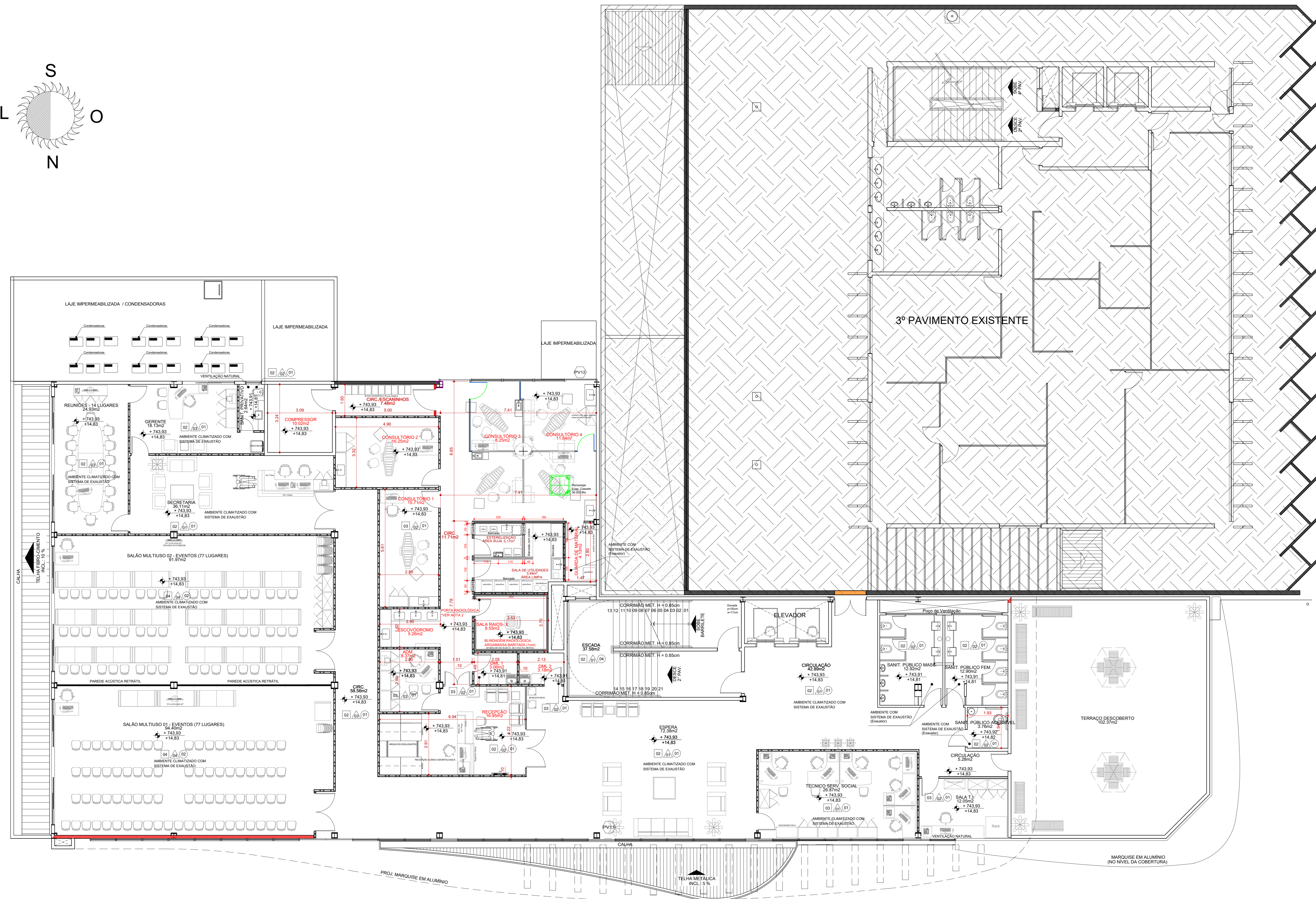
PLANTA LAYOUT 3º PAVIMENTO ESC.: 1/75
