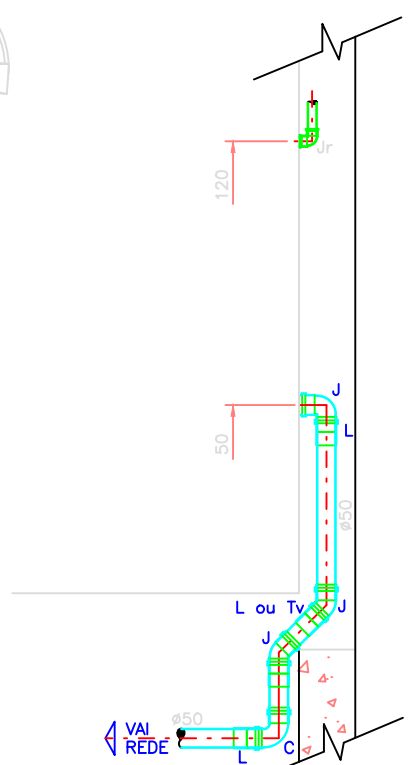
CORTE ESGOTAMENTO MICTÓRIO
