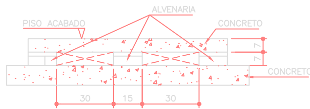
DETALHE CANALETA ESC. 1 : 20
