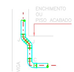
VISTA LATERAL LAVATÓRIO TANQUE
