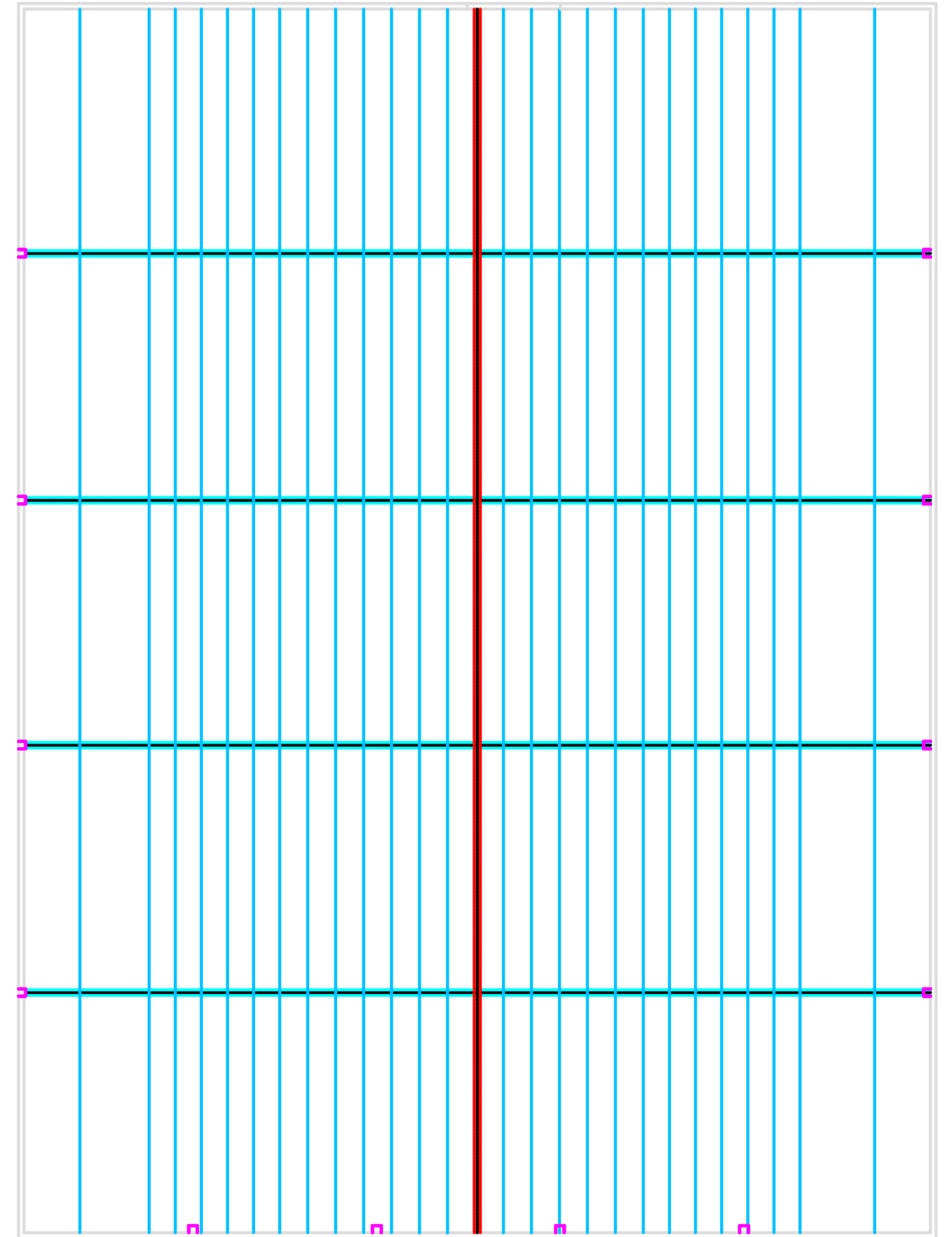
PLANO DE TERÇAS - QUADRA POLIESPORTIVA ESC.: 1:100
