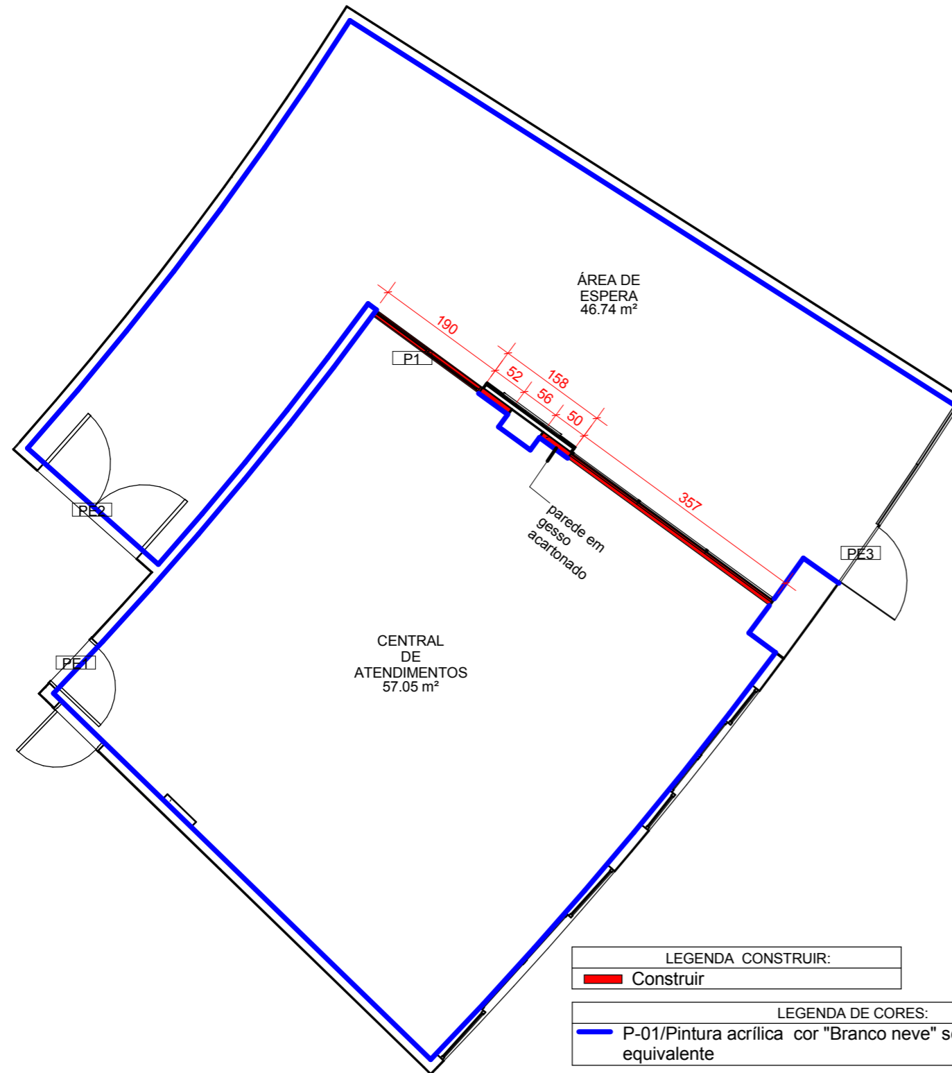
2 PLANTA RECEPÇÃO 1 : 75
