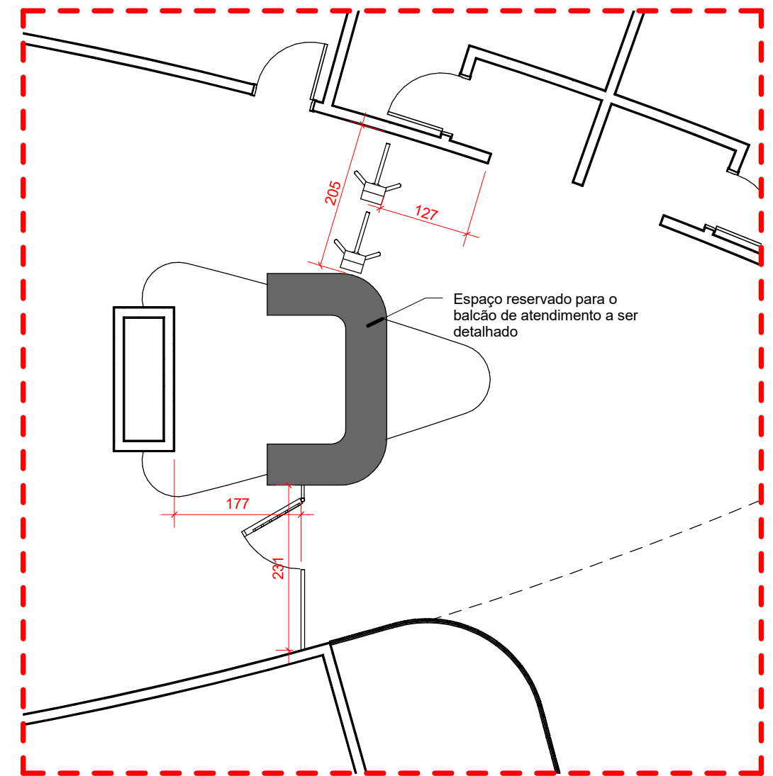
2 PLANTA BAIXA 1 : 75
