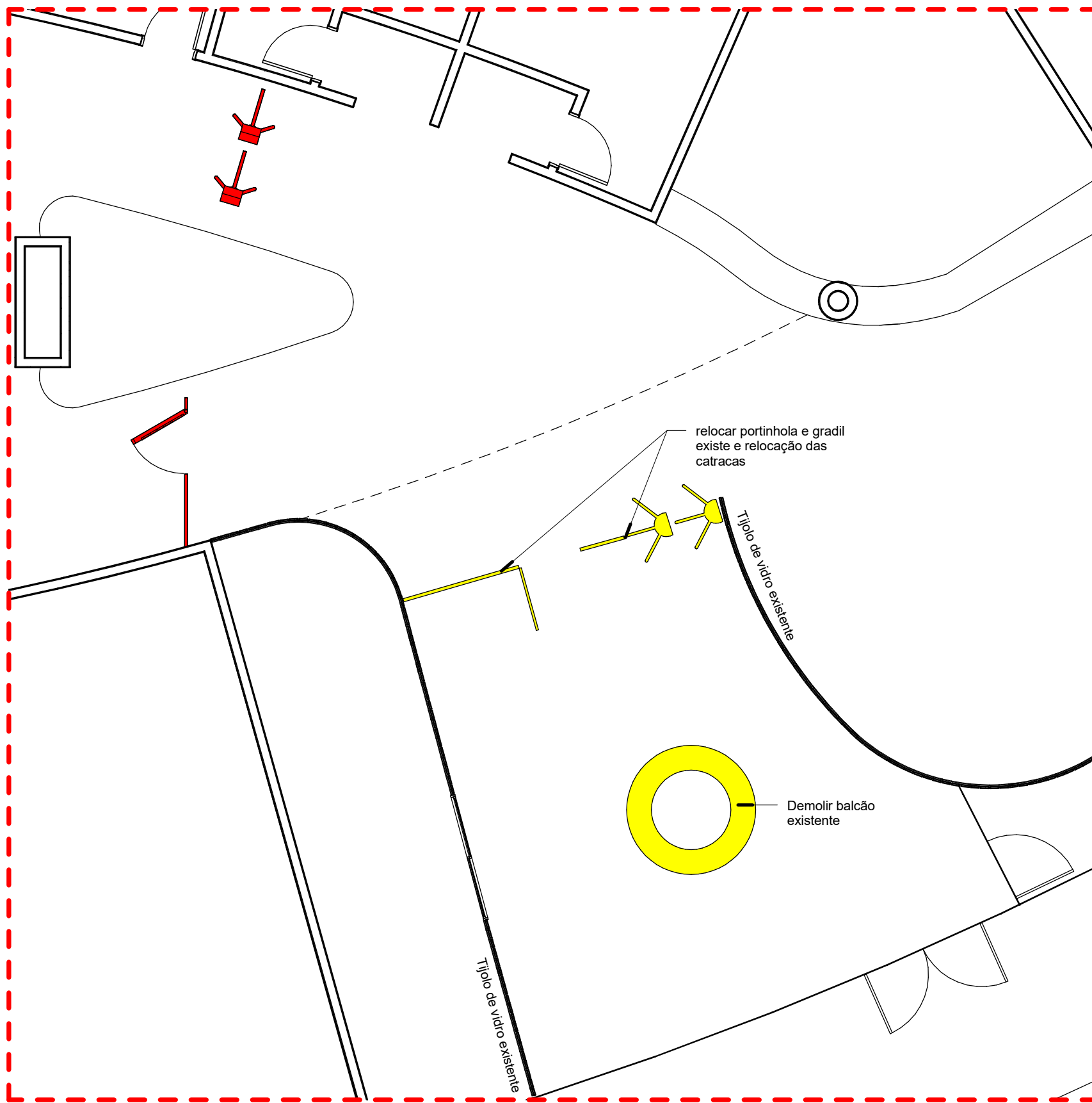
1 DEMOLIR E CONSTRUIR 1 : 75
