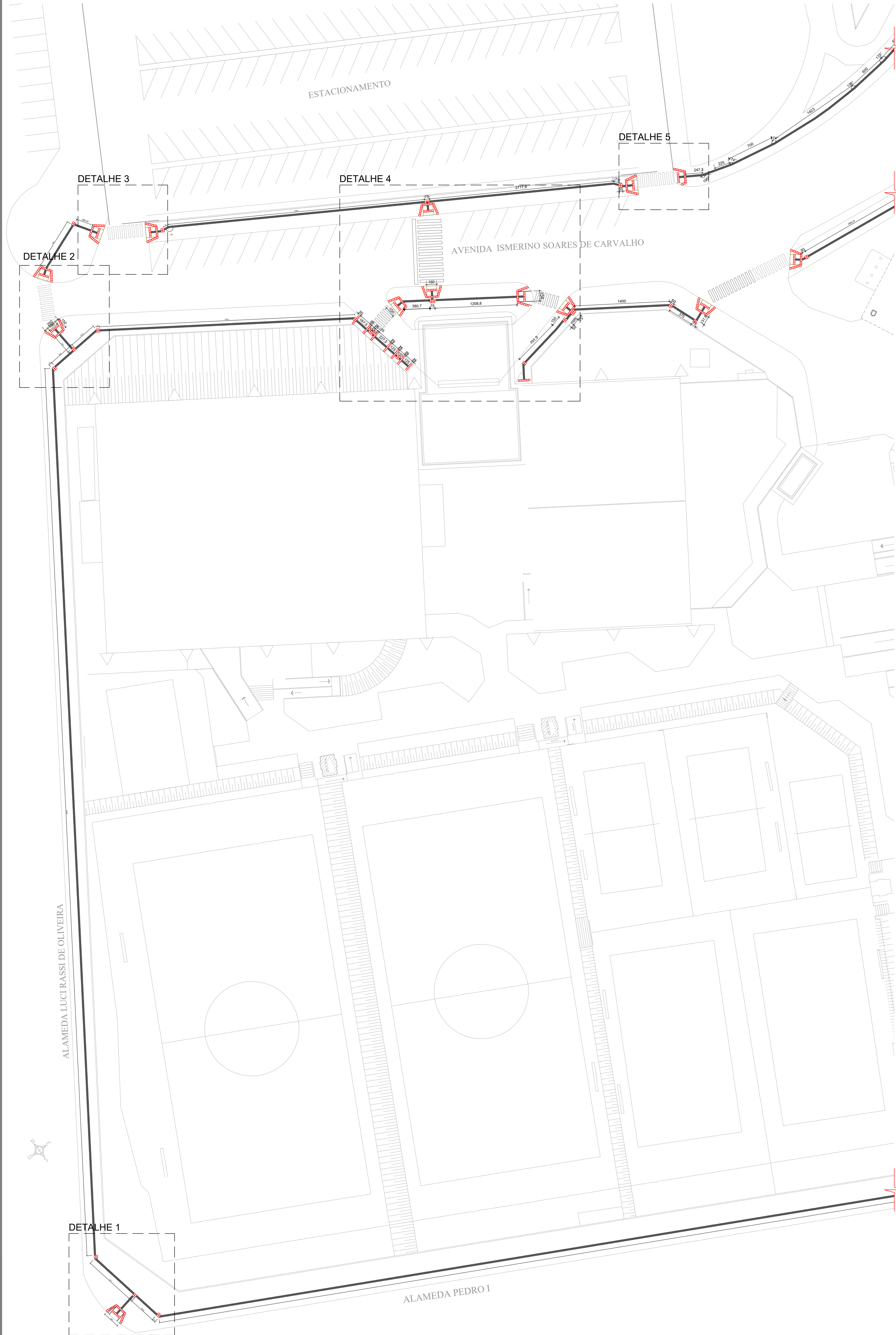
PLANTA TÉRREO DETALHES A- IMPLANTAÇÃO PISO TÁTIL ESCALA 1:250
