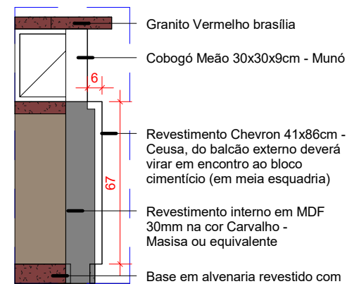
CORTE A ESC.: 1:20
