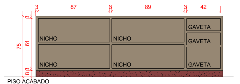
Det. 2 ARMÁRIO ESC.: 1 : 25
