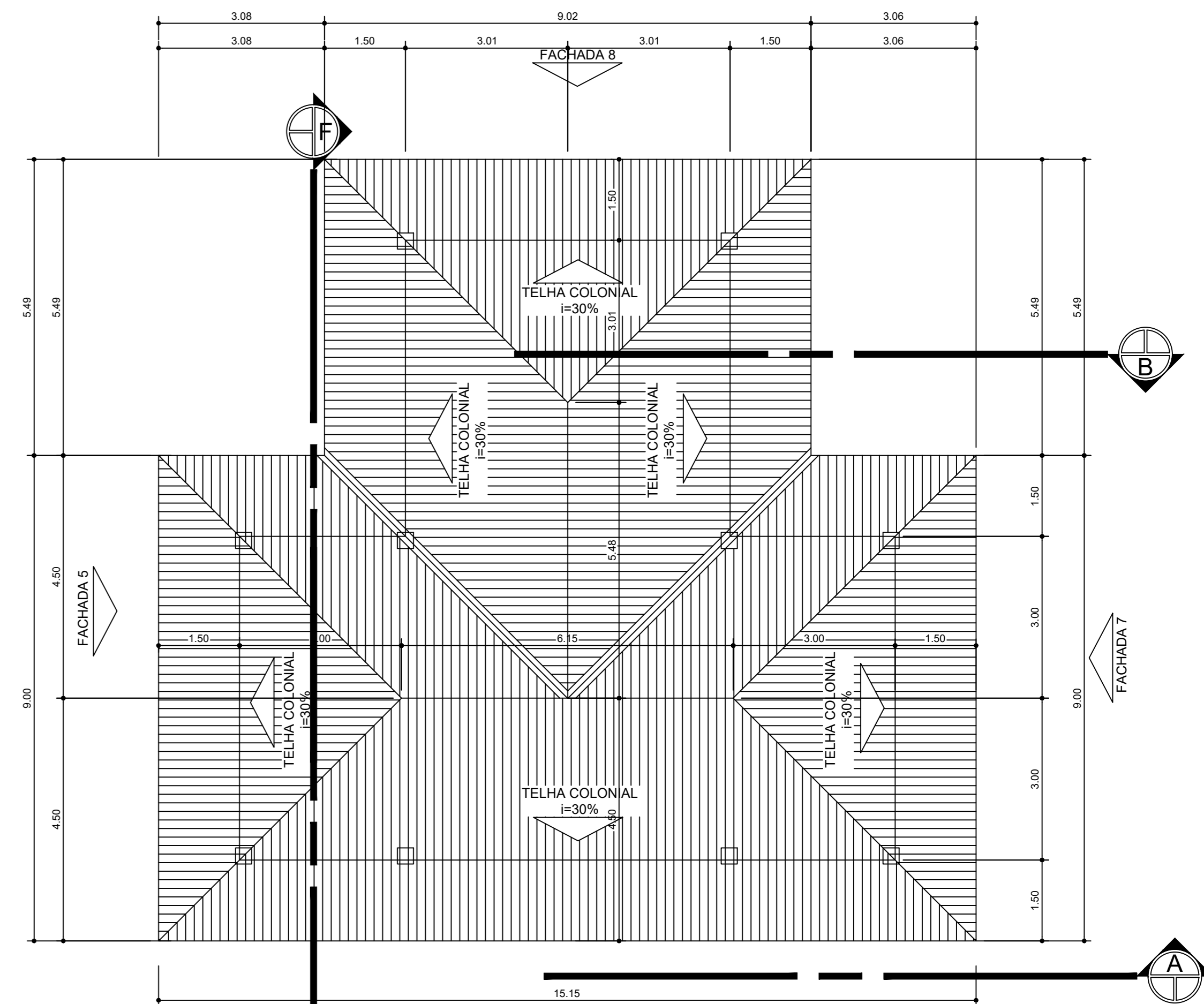
PLANTA COBERTURA - BLOCO A (ANEXO) ESC.: 1:75
