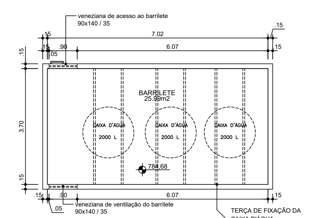
PLANTA BARRILETE - BLOCO A ESC.: 1:75
