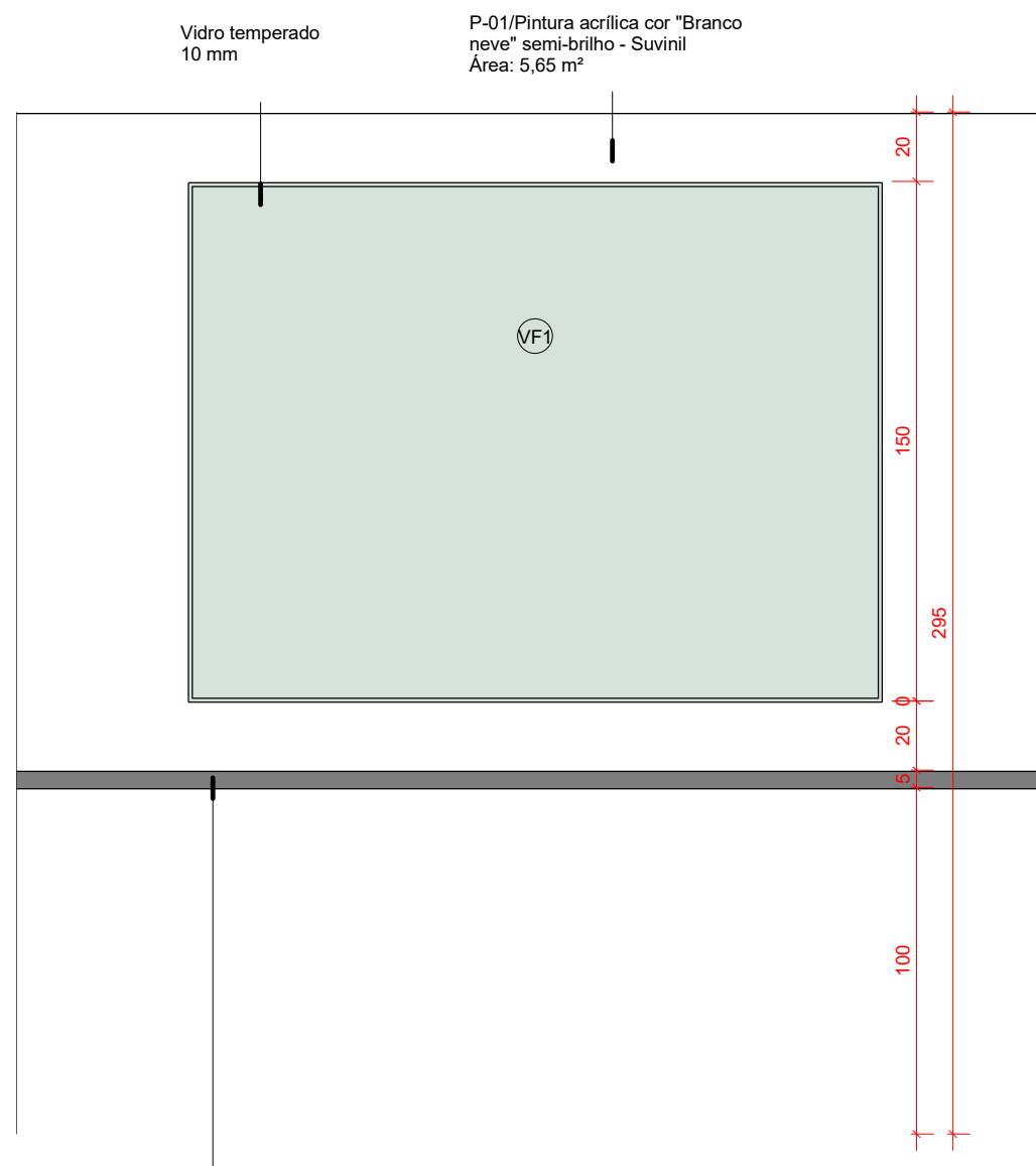
2 VISTA 5 1 : 20
