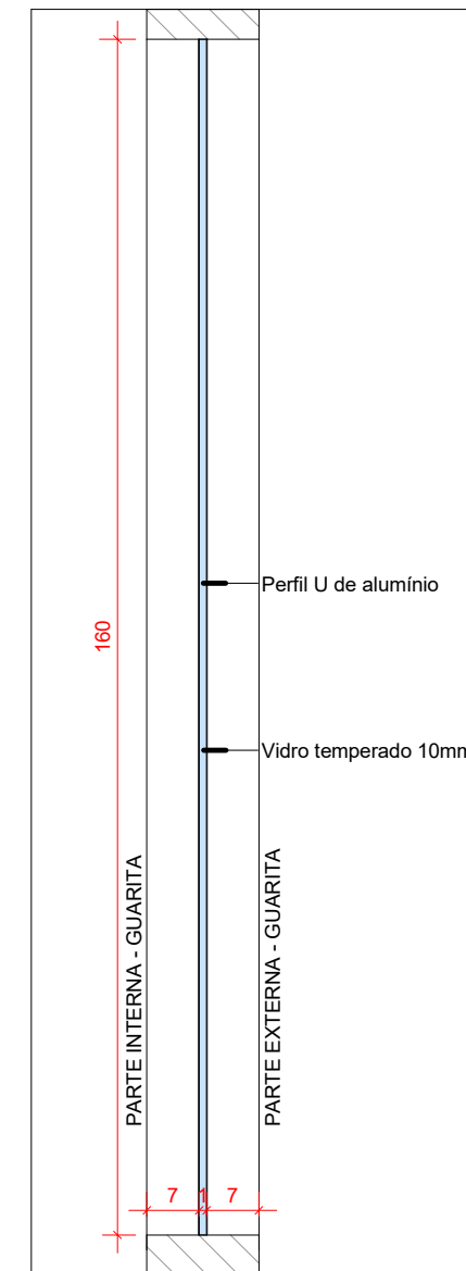
3 DETALHE VIDRO 1 : 10
