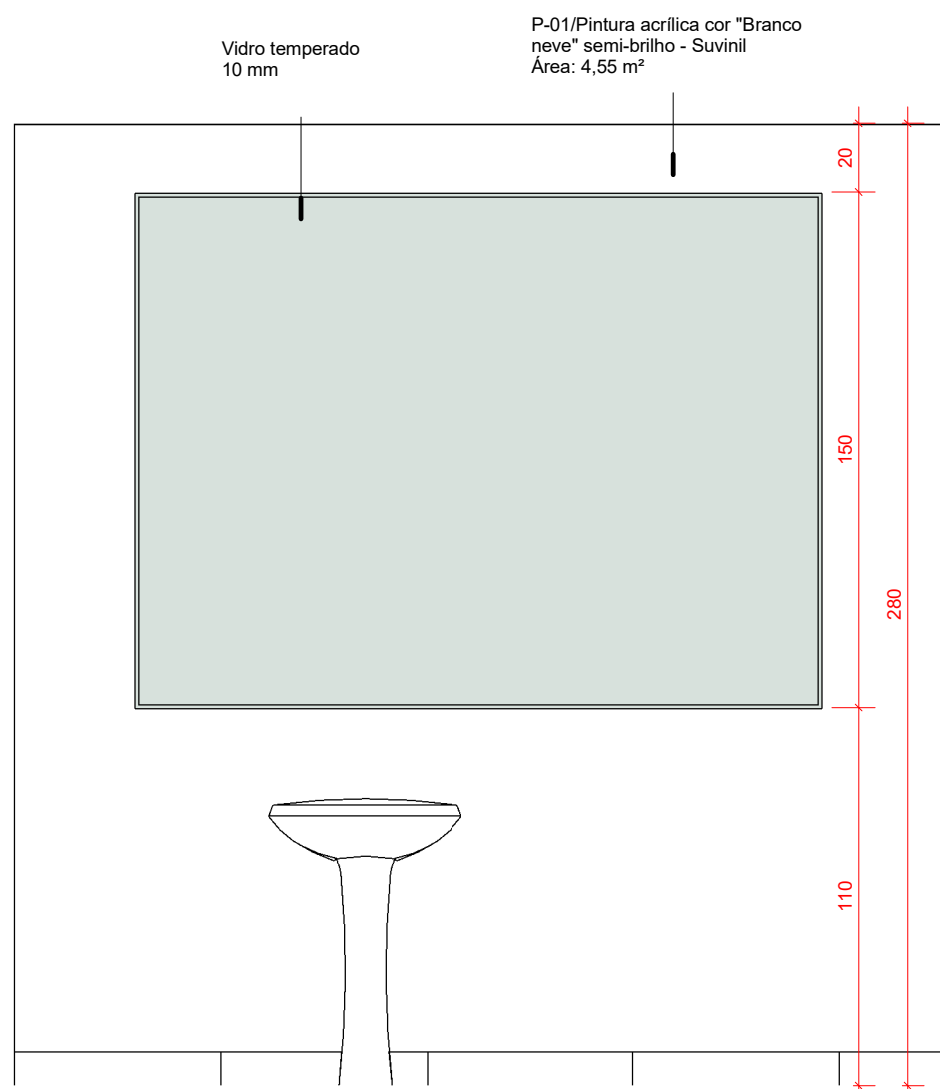
1 VISTA 4 1 : 20
