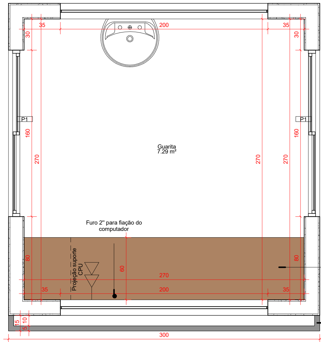
1 PLANTA LAYOUT 1 : 20
