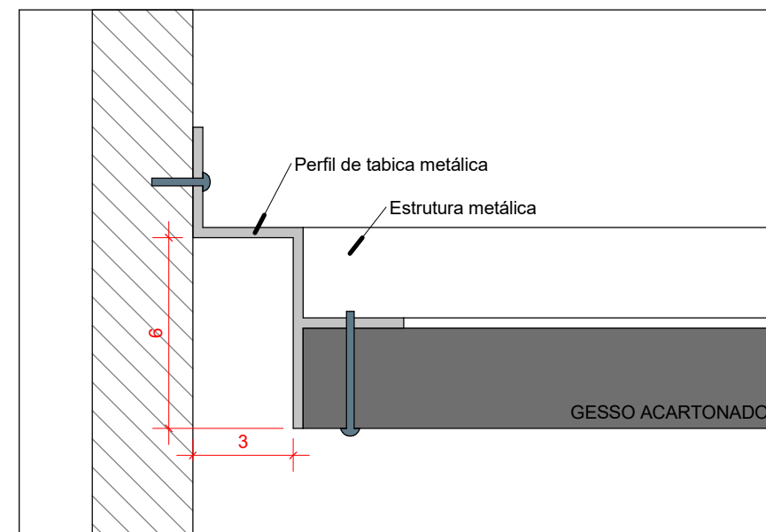
2 DET. 1 GESSO 1:2
