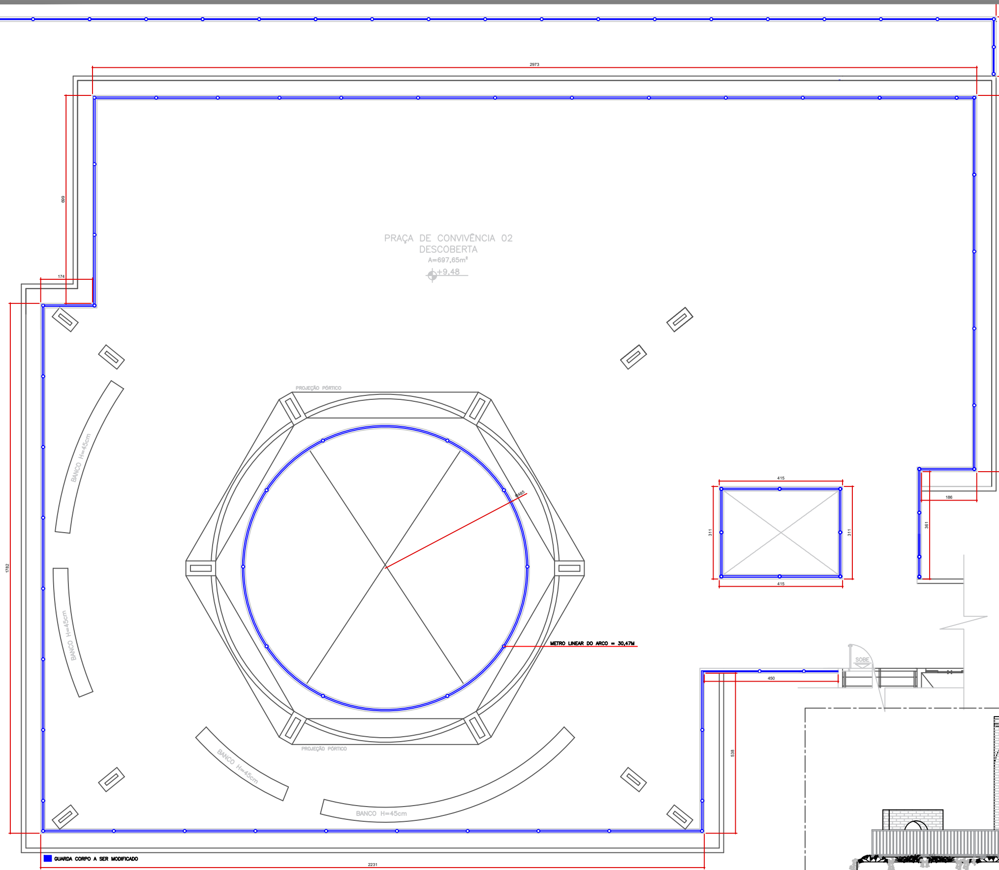
PLANTA BAIXA – GUARDA CORPO ESC. 1:125
