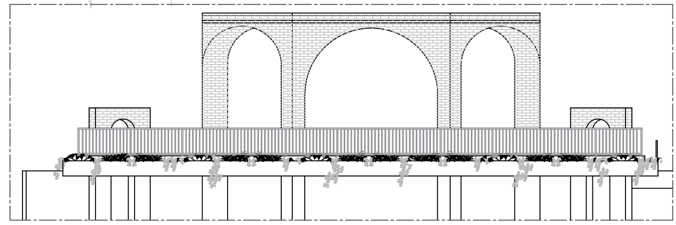
VISTA A ESC. 1:150
