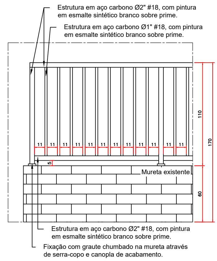
DETALHE GUARDA CORPO ESC. 1:25
