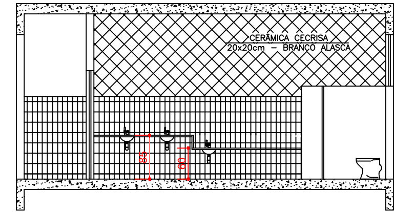
DETALHE 1 SANITÁRIOS- 1º PAVIMENTO ESC.: 1:75
