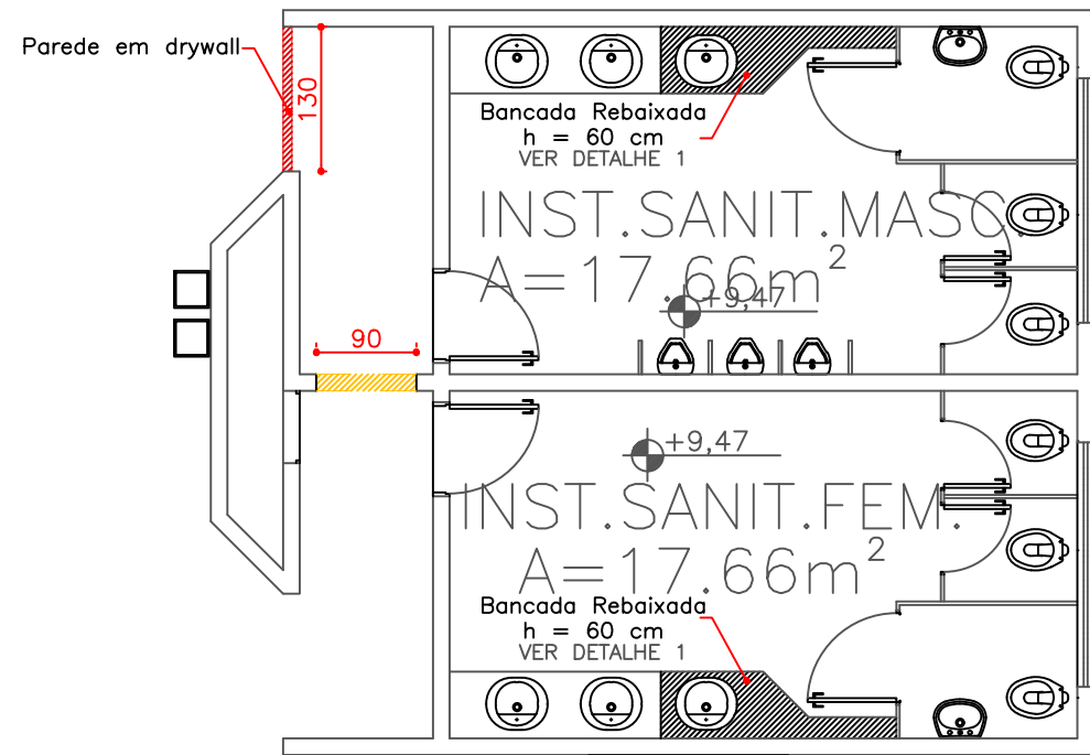
PLANTA CONSTRUIR E DEMOLIR SANITÁRIOS 1º PAVIMENTO ESC.: 1:75
