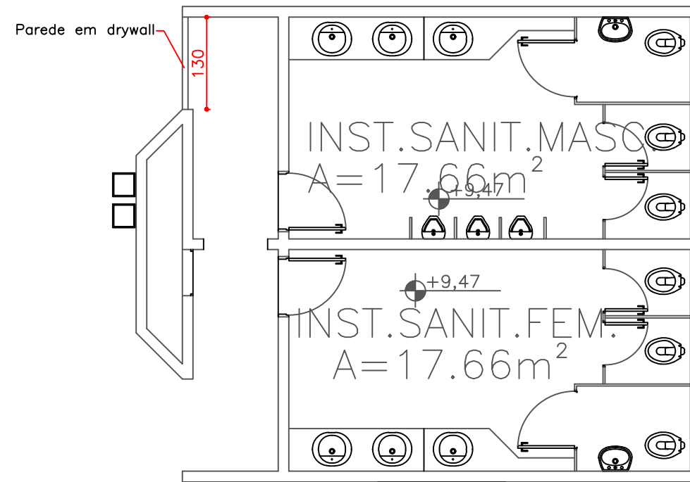
PLANTA MODIFICADA SANITÁRIOS 1º PAVIMENTO ESC.: 1:75
