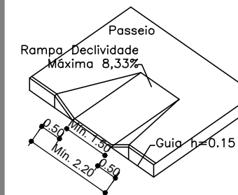
DETALHE 2- REBAIXO DE MEIO FIO RAMPA PCD (PADRÃO SMT) SEM ESCALA
