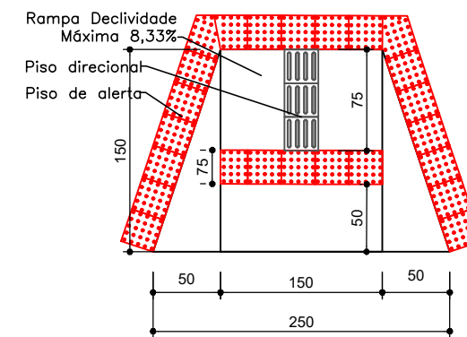
DETALHE 1- REBAIXO DE MEIO FIO RAMPA PCD (PADRÃO SMT) SEM ESCALA
