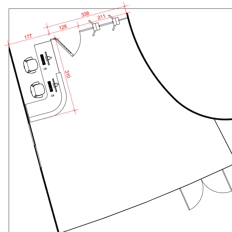
2 PLANTA BAIXA 1 : 75
