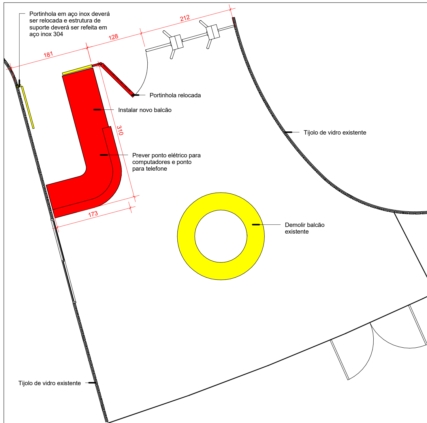
1 DEMOLIR E CONSTRUIR 1 : 50
