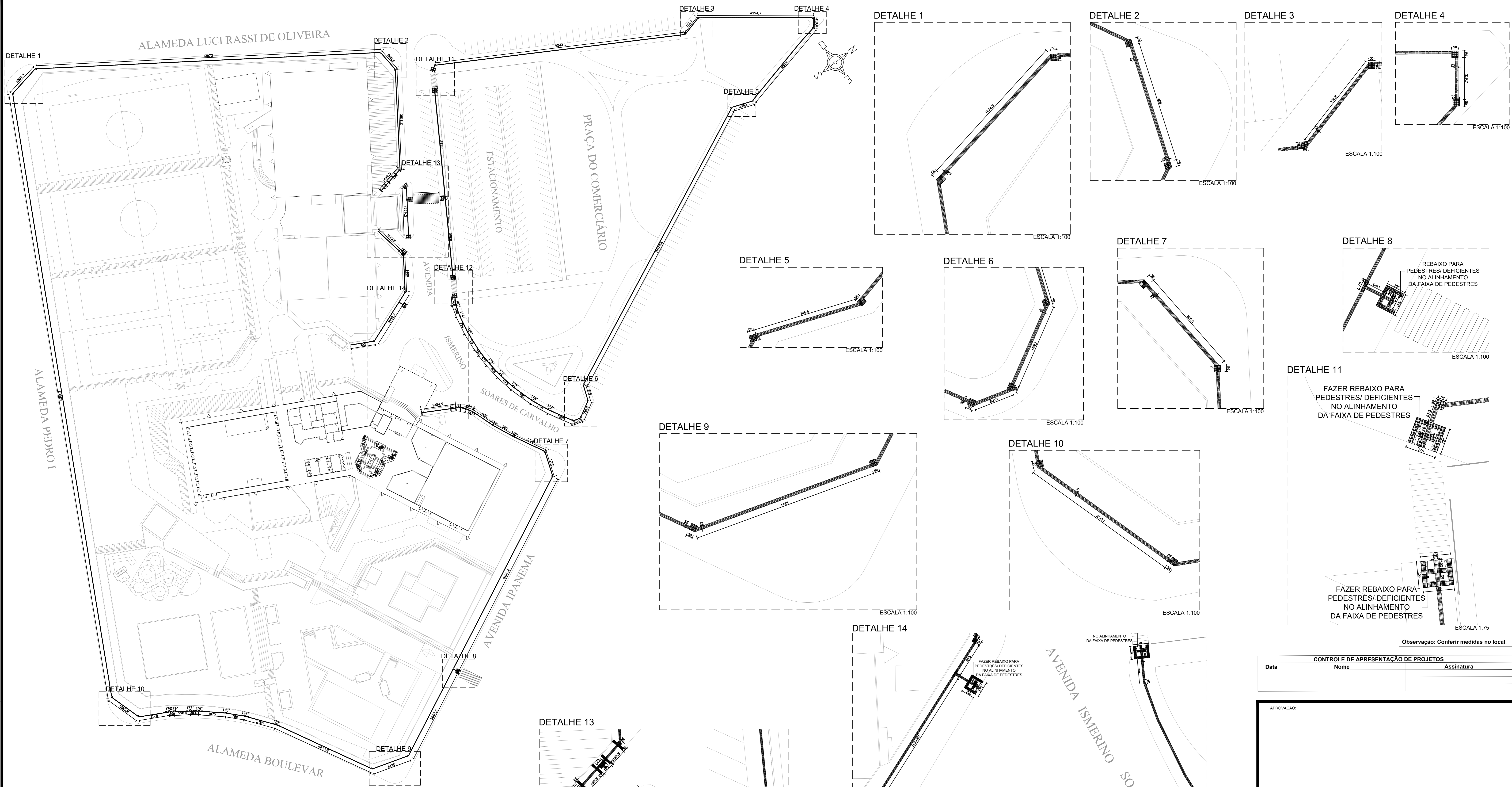
PLANTA TÉRREO - IMPLANTAÇÃO PISO TÁTIL ESCALA 1:500
