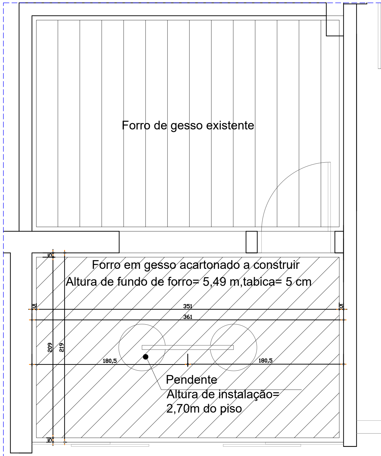
PLANTA DE FORRO ESC.1:25
