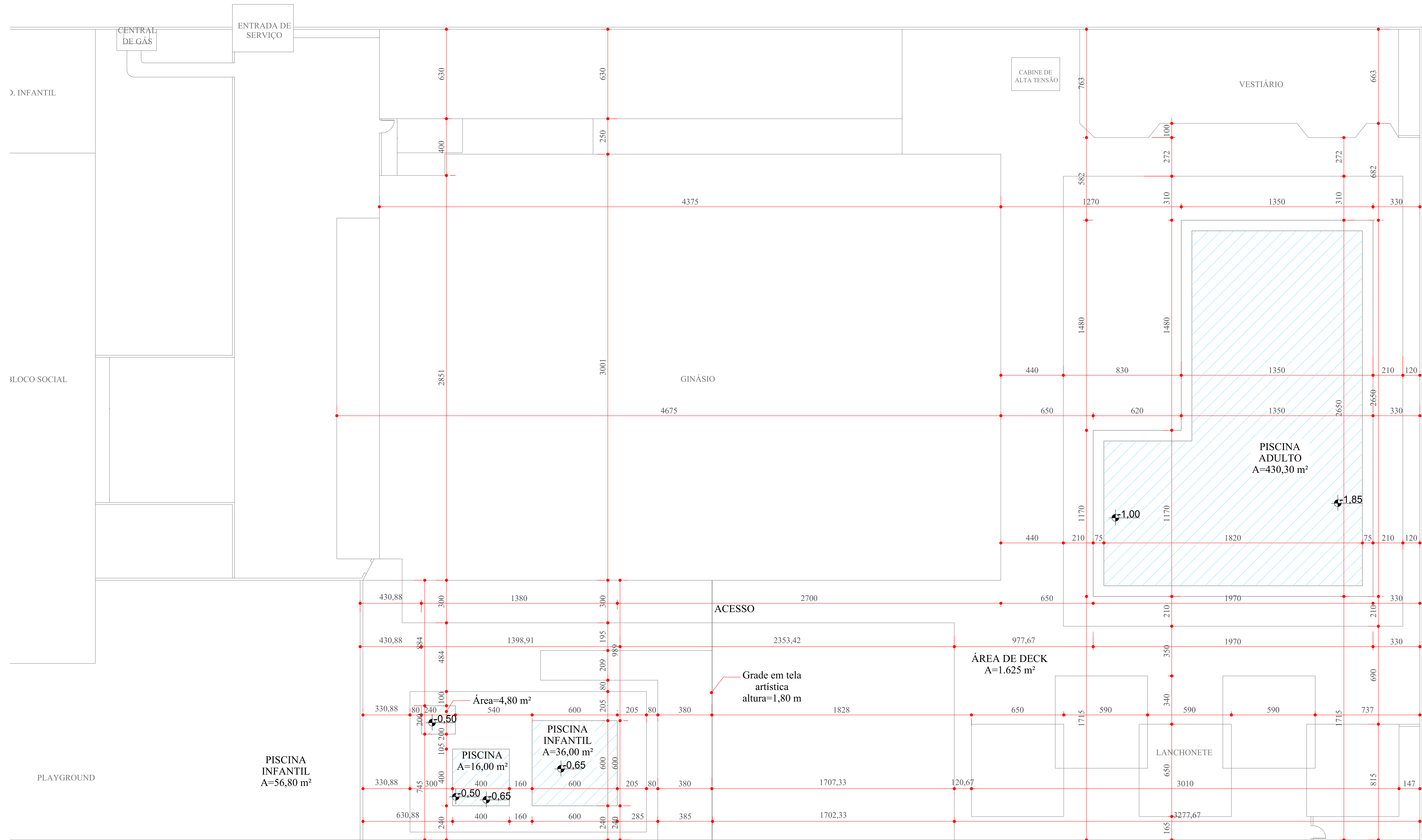
PLANTA IMPLANTAÇÃO ESCALA 1:250
