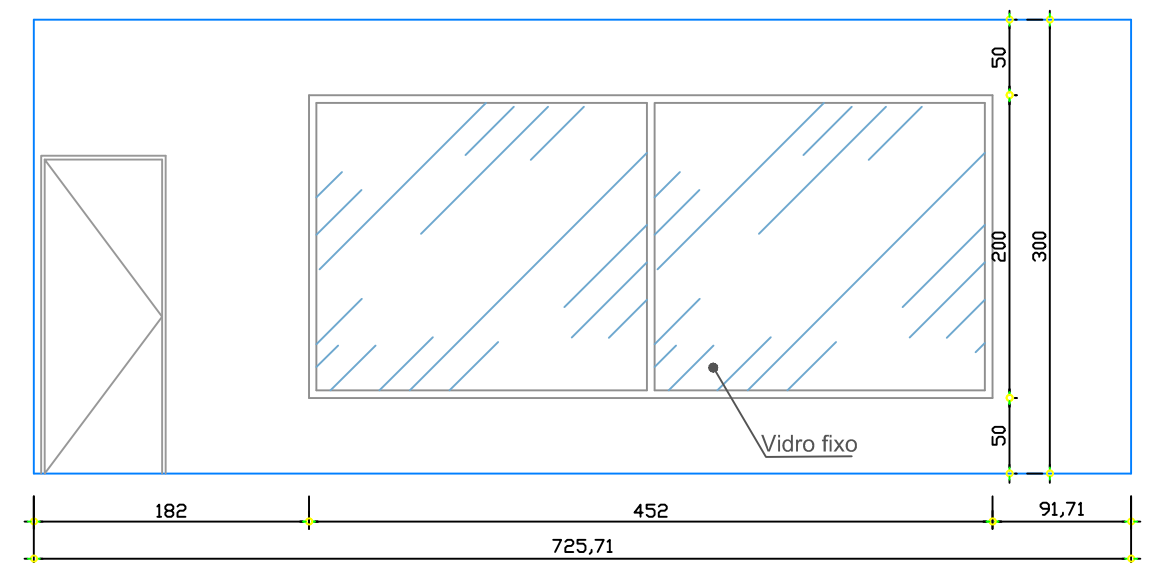
VISTA 4 ESC.1:50
