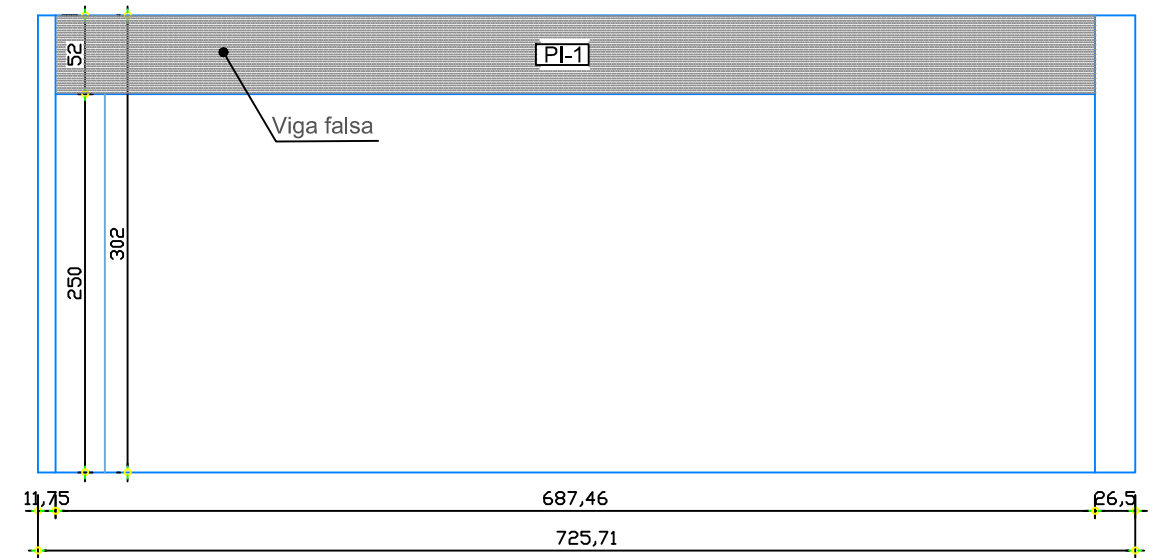
VISTA 2 - VISTA MODIFICADA ESC.1:50
