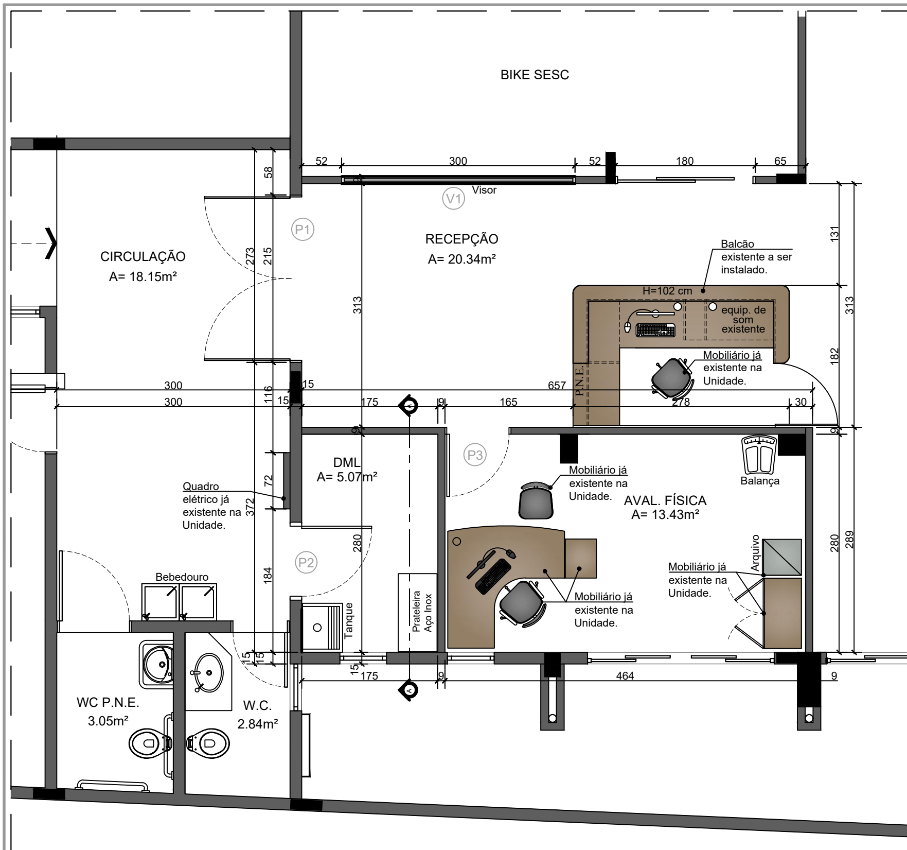
PLANTA LAYOUT ESCALA 1:50
