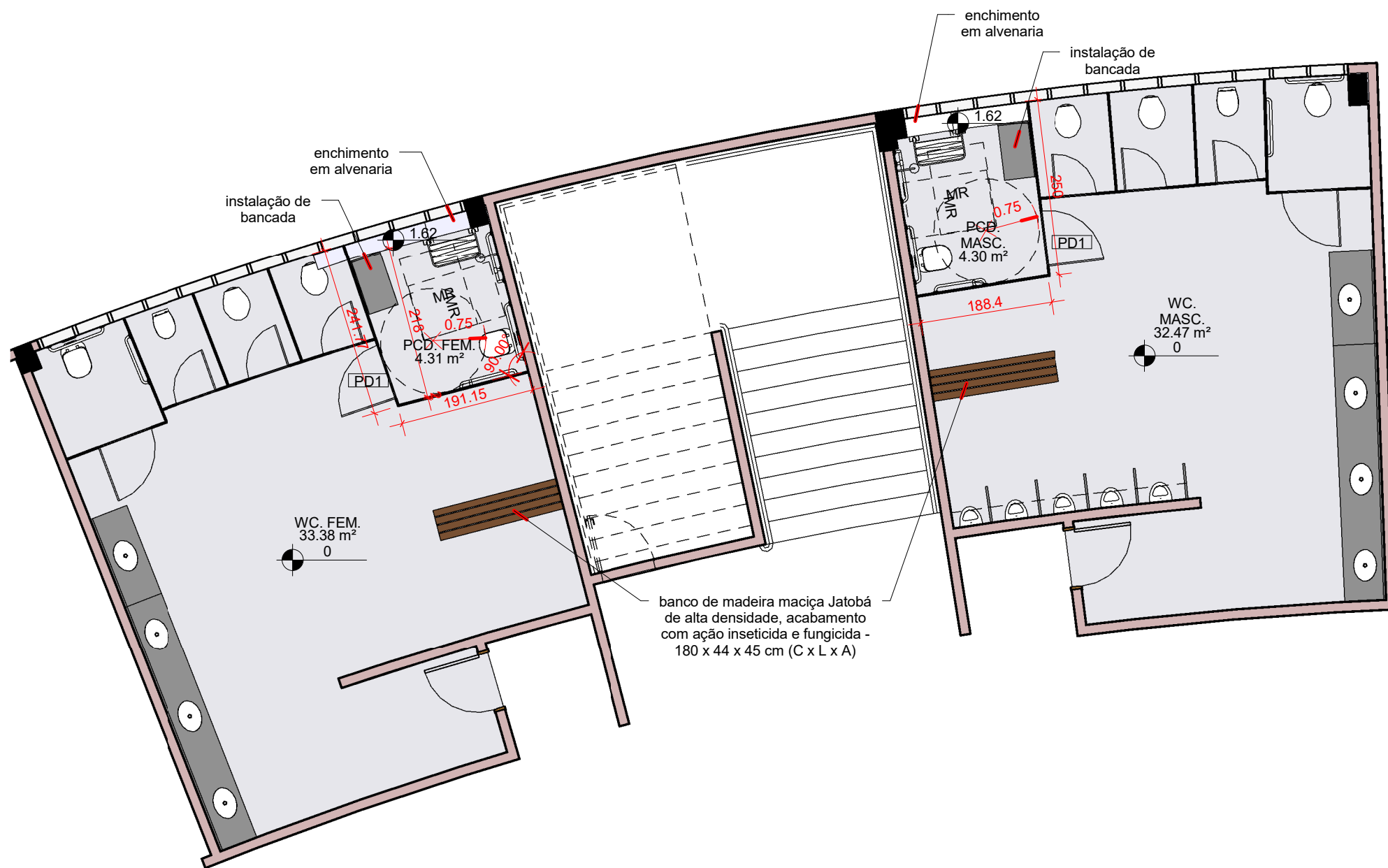
1 PLANTA 1 : 75
