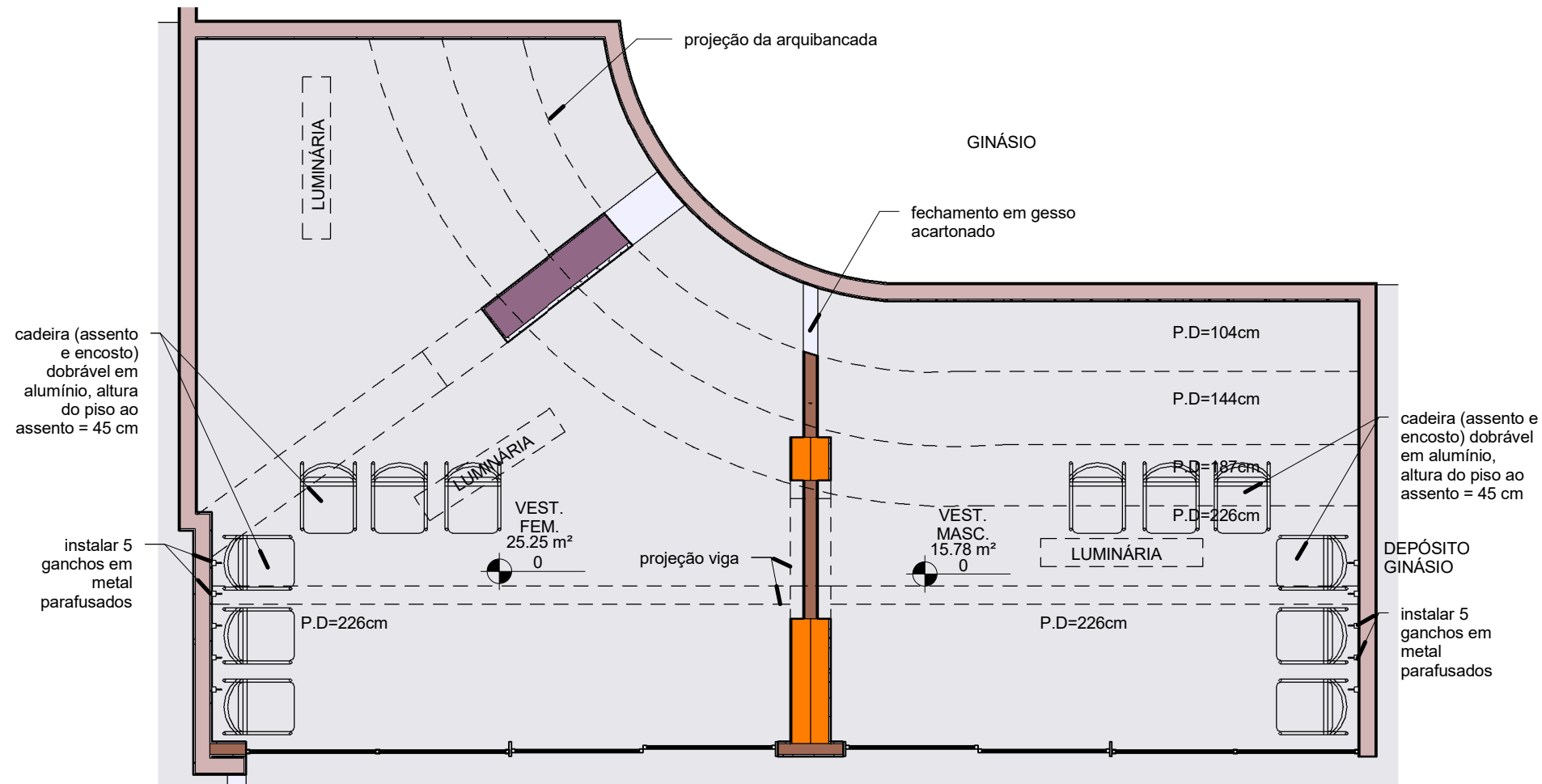
1 PLANTA VESTIÁRIO - LAYOUT 1 : 50
