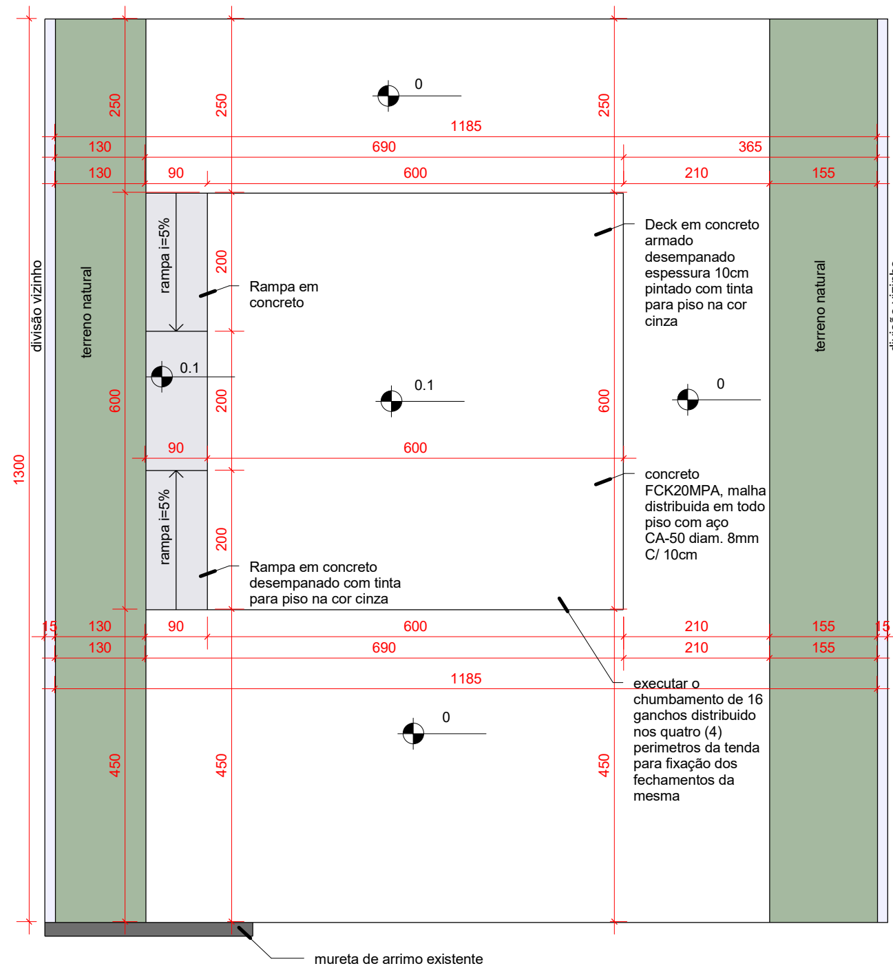
1 DECK 1 : 75
