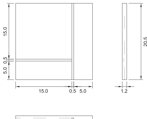
PVC ou MDF vistas ortográficas
