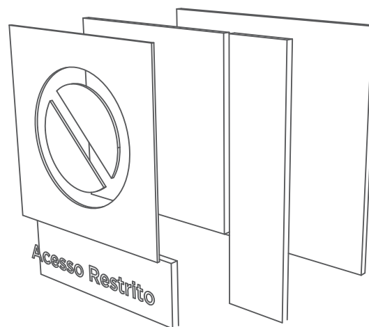
Peças completas vista esquemática explodida
