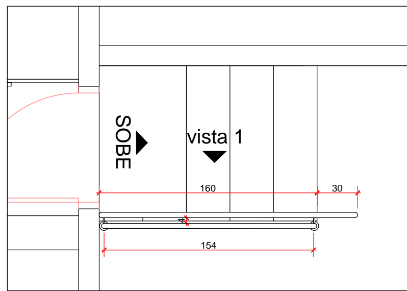
planta baixa
