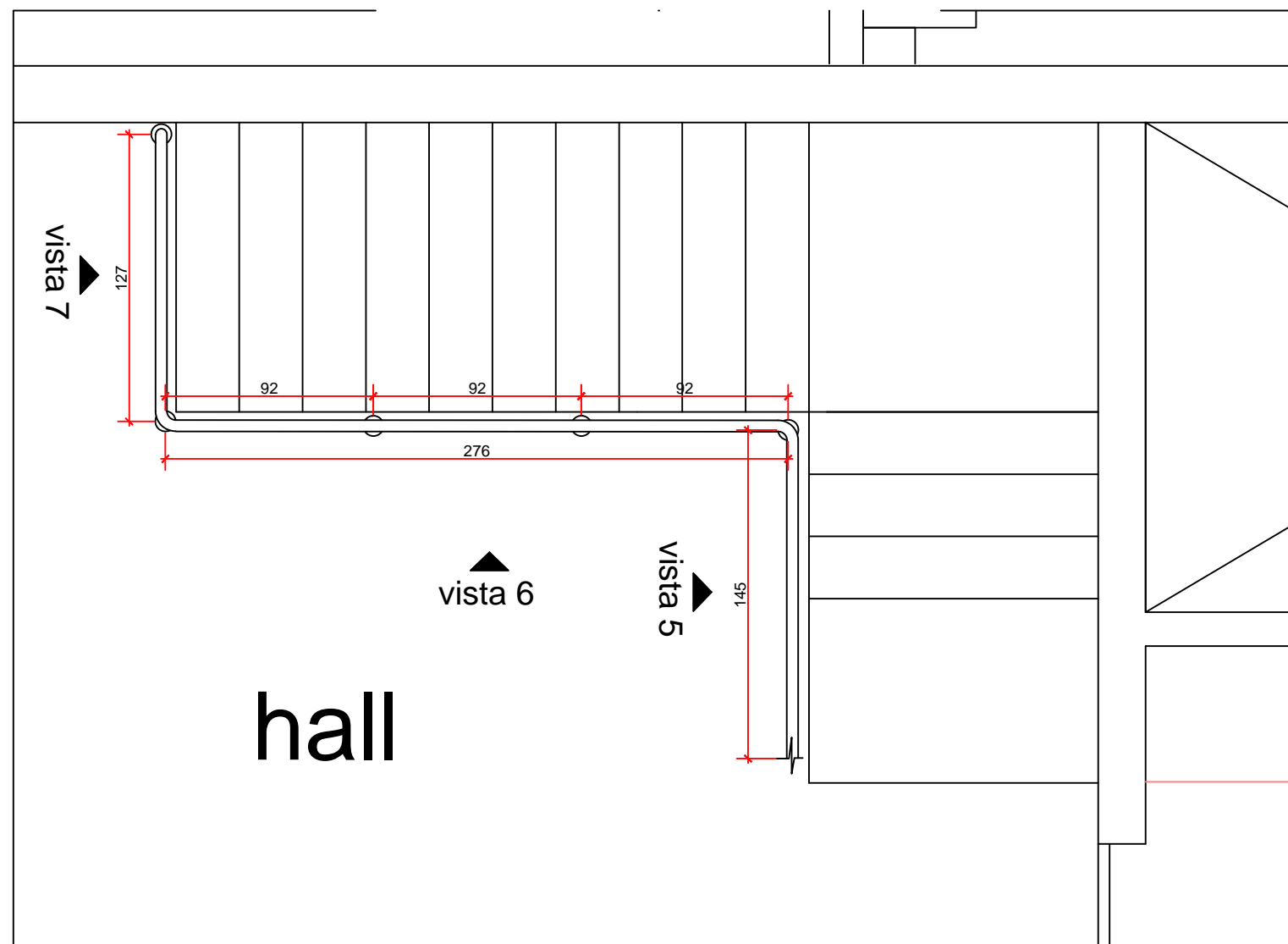
planta baixa - escada 1º pavimento
