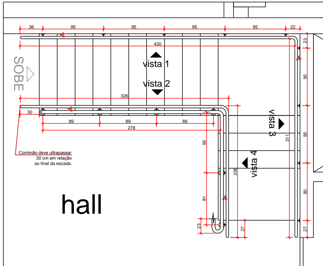
planta baixa - térreo escada
