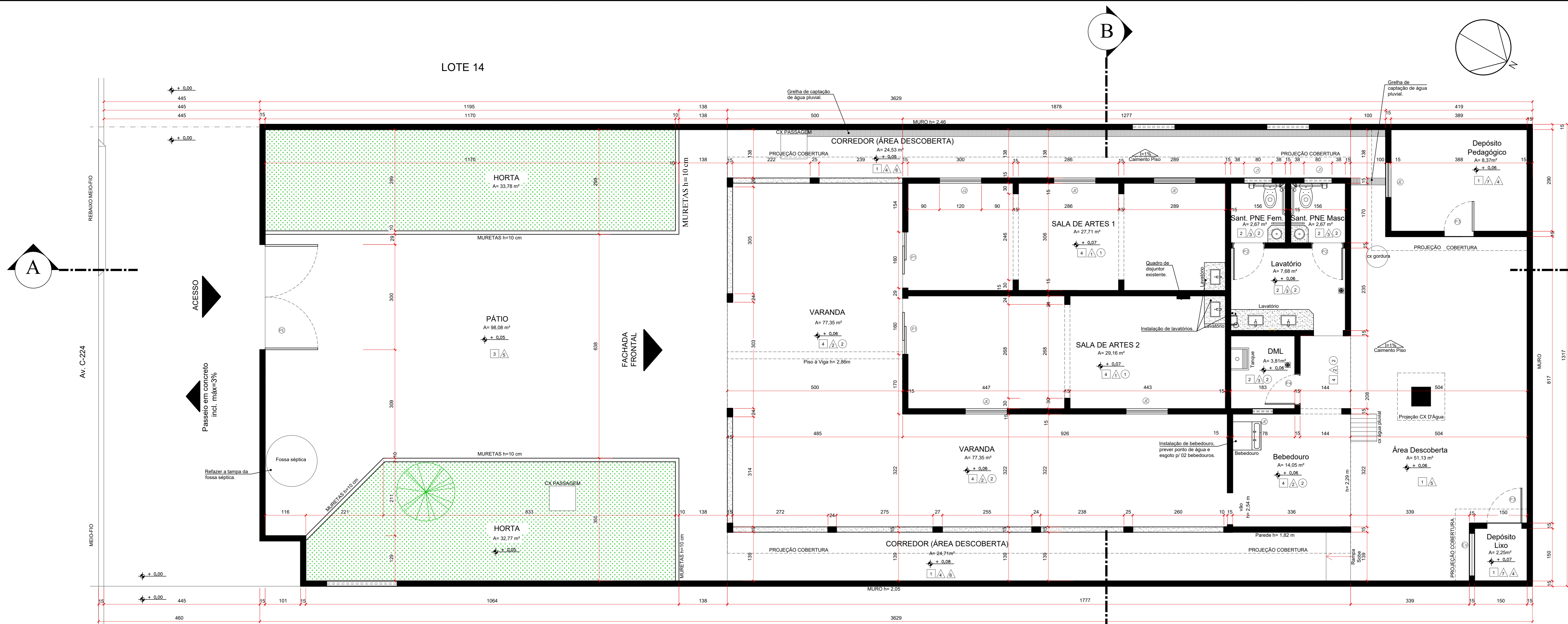
PLANTA TÉRREO/IMPLANTAÇÃO ESC 1/50
