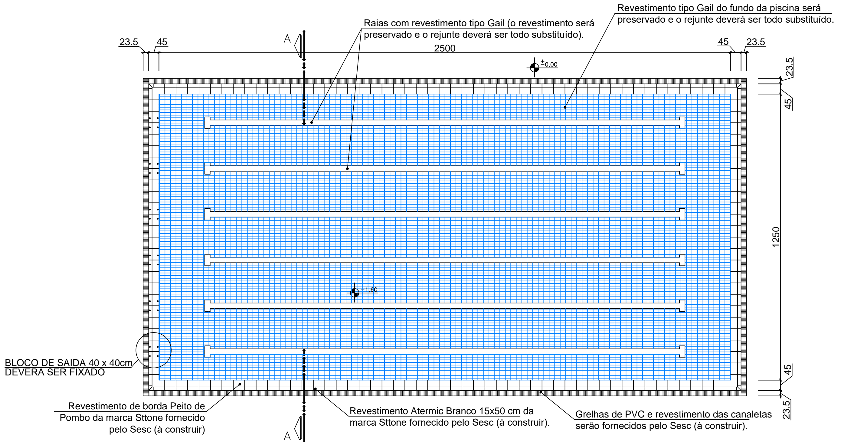
VISTA SUPERIOR ESC.:1:100
