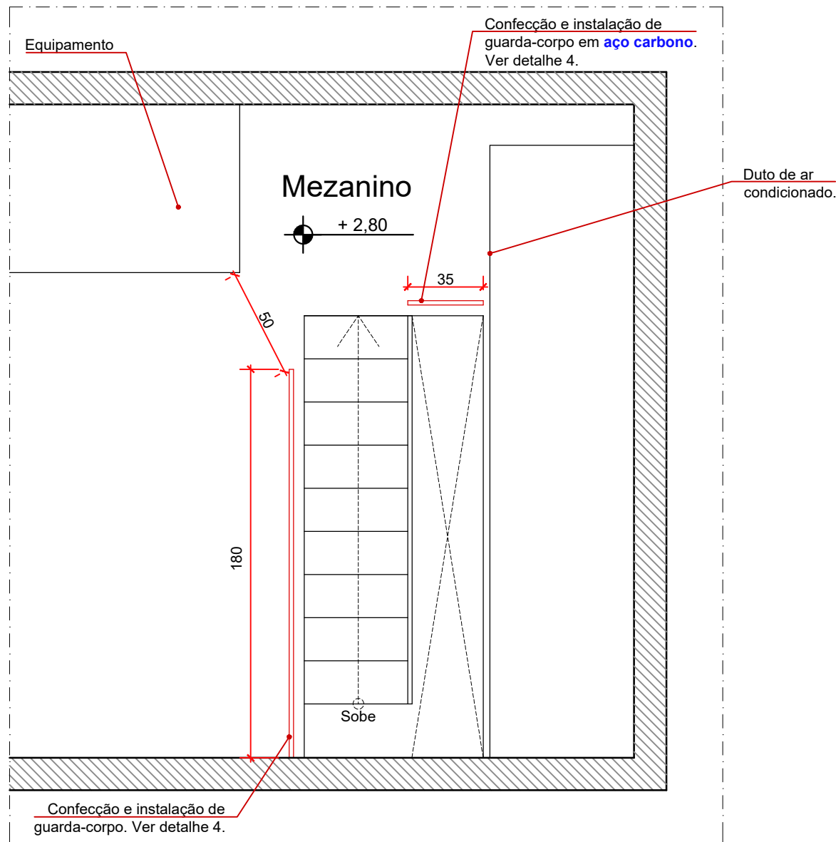
PLANTA SALA DE MÁQUINAS - AUDITÓRIO esc.: 1/25
