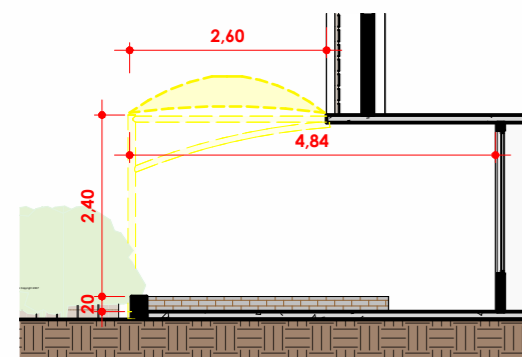
3 CORTE A ESCALA 1:100
