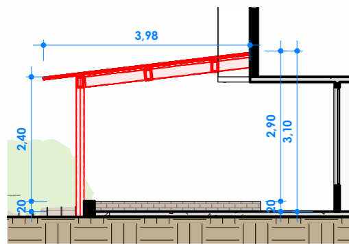
3 CORTE B ESCALA 1 : 100
