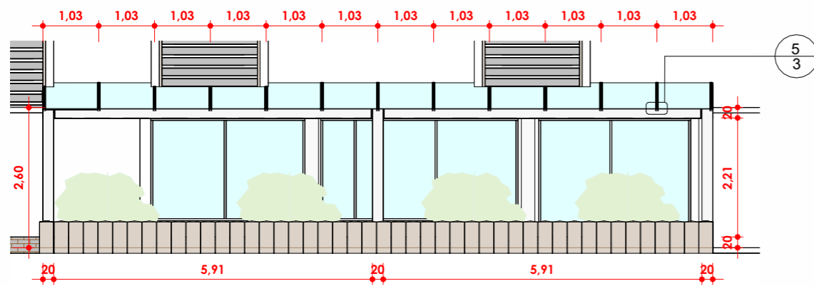
2 VISTA FRONTAL ESCALA 1 : 100
