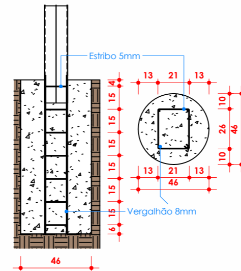
6 DETALHE ESTACA ESTRUTURAL ESCALA 1 : 25
