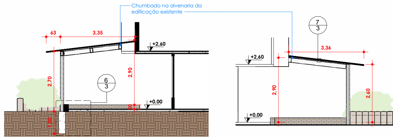
3 CORTE C ESCALA 1 : 100
