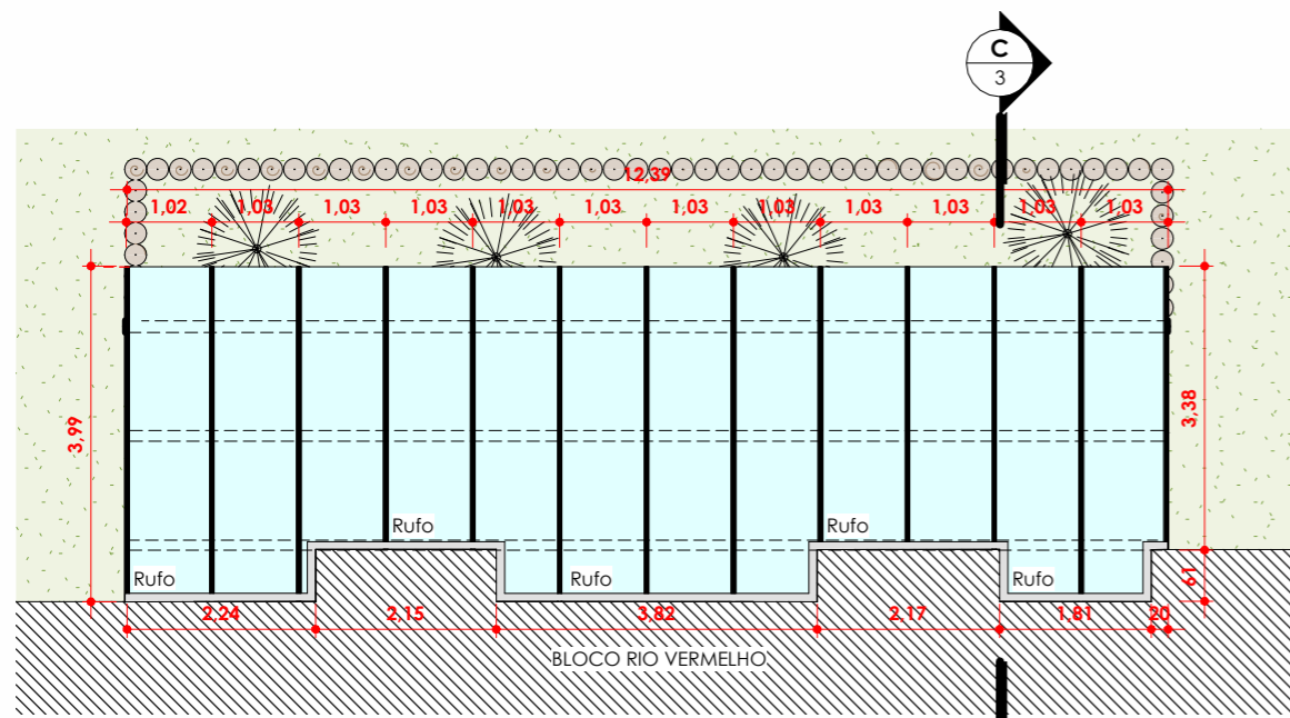
1 PLANTA DE LOCAÇÃO E COBERTURA ESCALA 1 : 100
