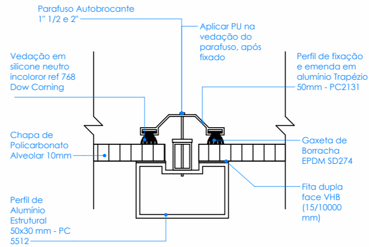
5 DETALHE JUNTA ALUMÍNIO ESCALA 1 : 50
