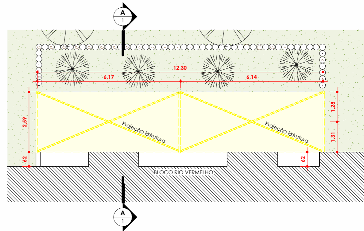
5 PLANTA DE LOCAÇÃO E COBERTURA ESCALA 1:100
