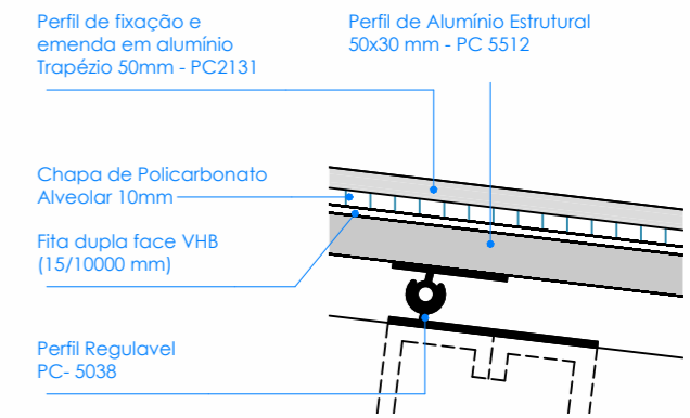
7 DETALHE PERFIL REGULÁVEL ESCALA 1 : 5
