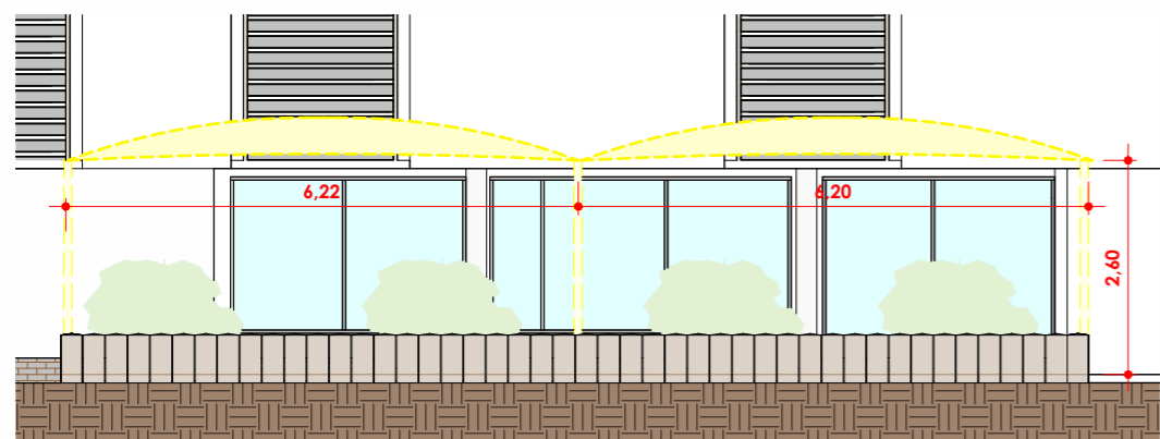
2 VISTA FRONTAL ESCALA 1:100
