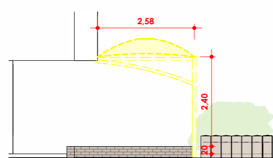
4 VISTA LATERAL ESCALA 1:100
