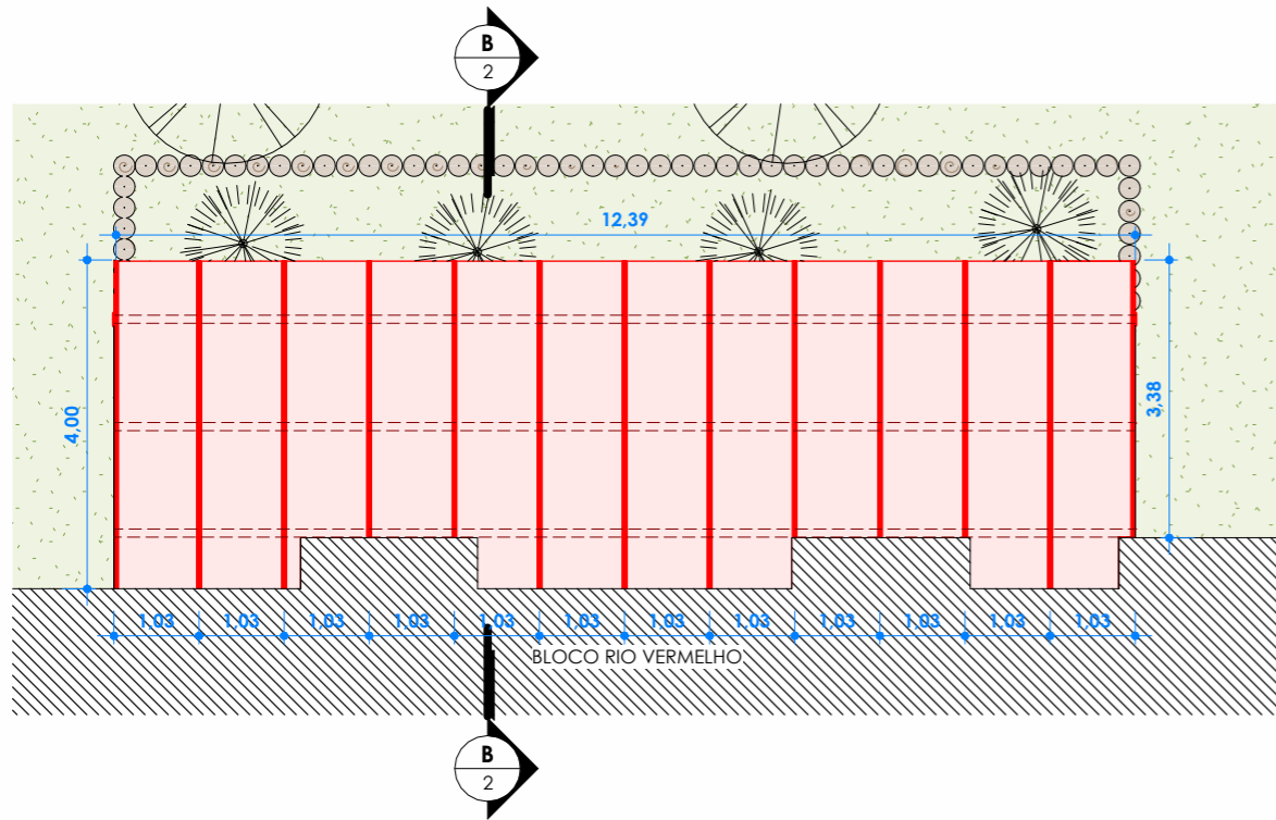
1 PLANTA DE LOCAÇÃO E COBERTURA ESCALA 1 : 100
