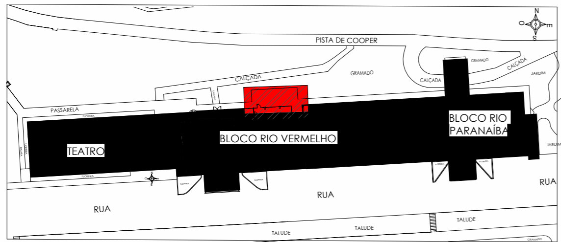
1 IMPLANTAÇÃO ESCALA 1:1000
