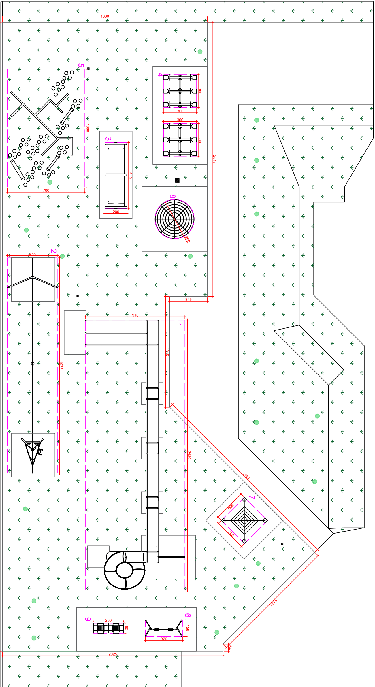
Sesc Falcatville - Parque Infantil - Recreação 1:150
