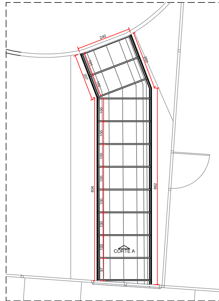
Planta de Cobertura de Policarbonato Esc. 1:100
