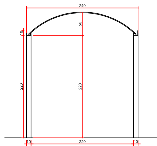
Corte A Esc. 1:50
