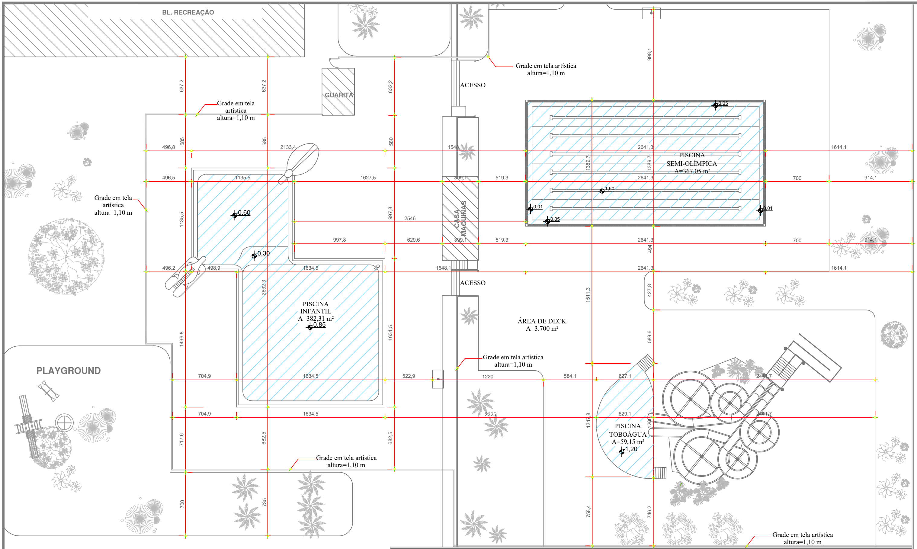
PLANTA IMPLANTAÇÃO ESCALA 1:250
